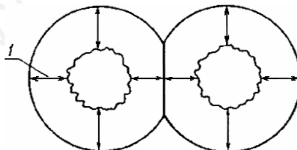
I - минимальная толщина Черт. 11
