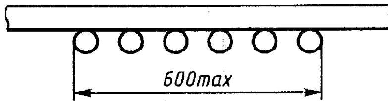
Рисунок 36 — Несоприкасающиеся кабели, закрепленные на передней стороне широкой лестницы (A (F) > 35 мм 2 )
