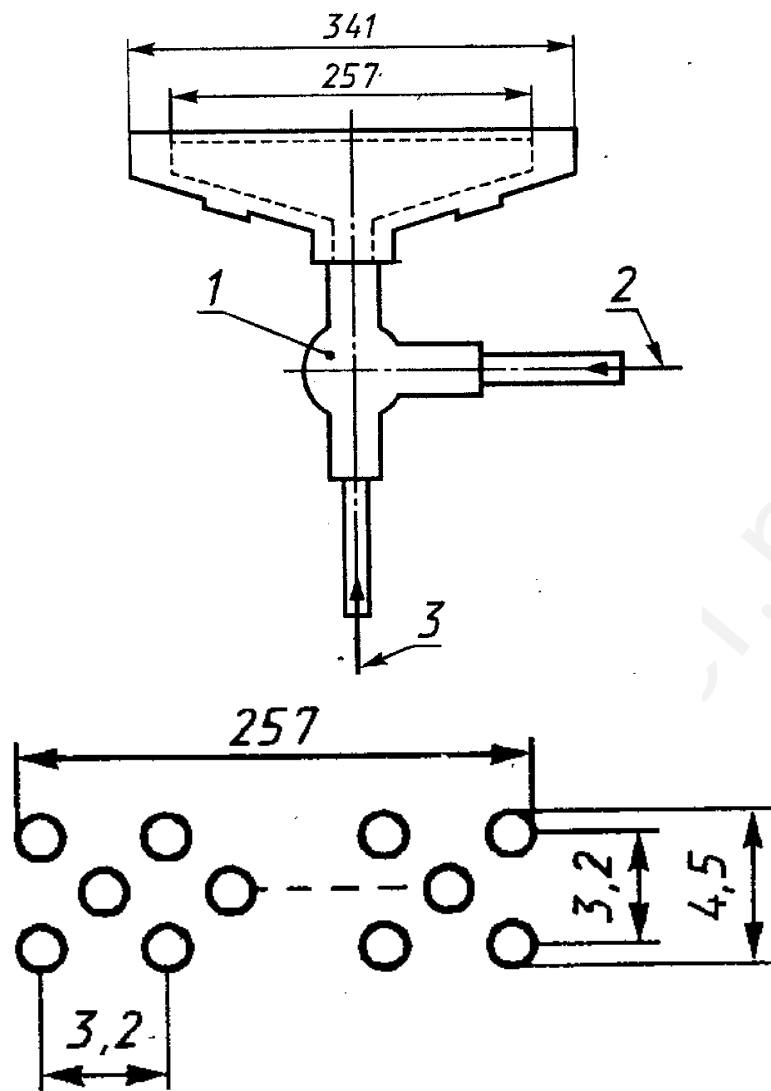
Рисунок 4 — Горелка
