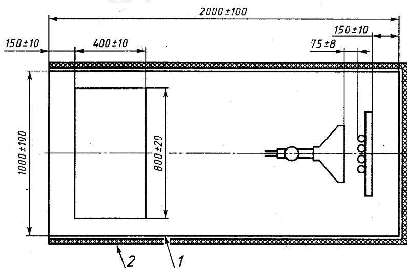
Рисунок 1 — Испытательная установка
