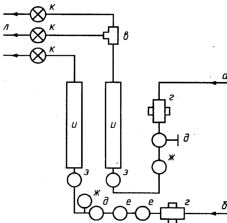
Рисунок 4а — Сдвоенная горелка
