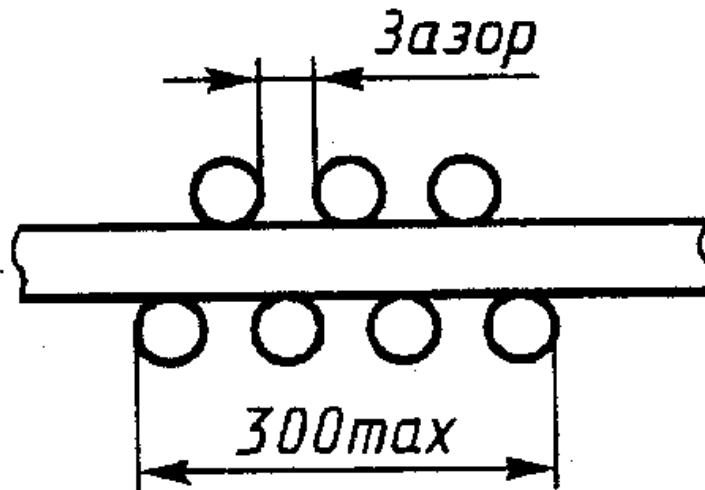
Рисунок 36 — Несоприкасающиеся кабели, закрепленные на передней стороне широкой лестницы (A (F) > 35 мм 2 )
